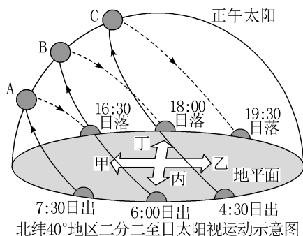
北纬40°地区二分二至日太阳视运动示意图
